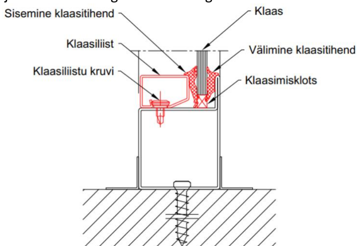
Joonis 9 Klaasi paigaldus
