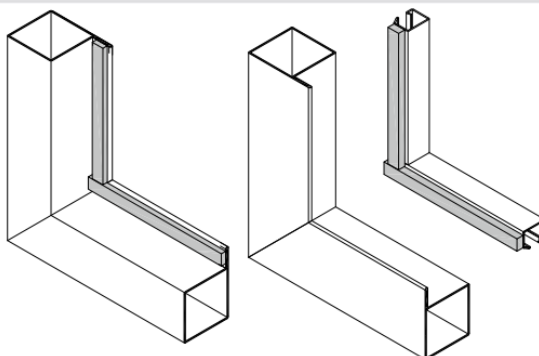
Joonis 10 Nelikanttihendi paigaldus
