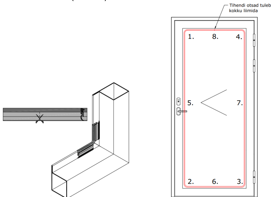
Joonis 7 Välimise klaasitihendi paigaldus
