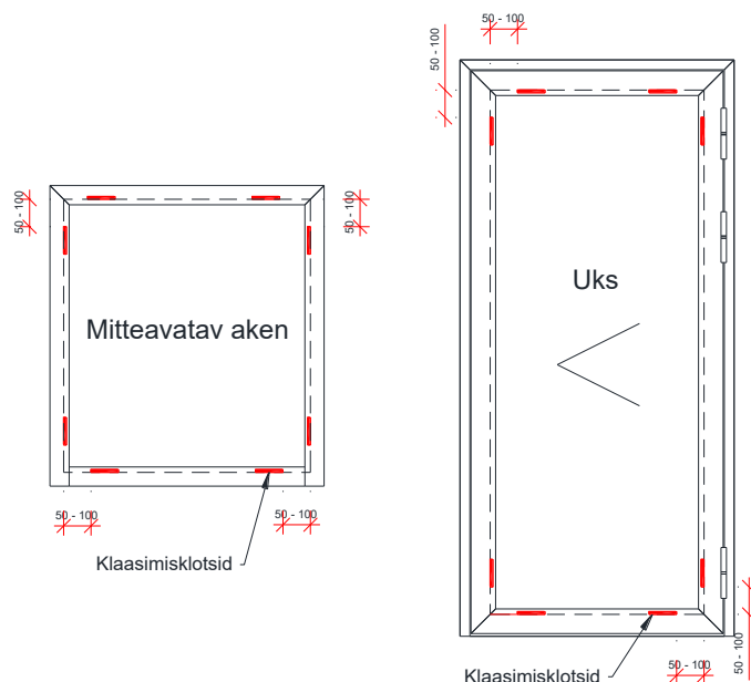
Joonis 6 Klaasimisklotside asukohad
