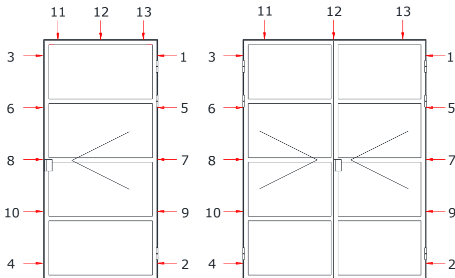
Joonis 2 Seinakinnituste järjekord uksele
