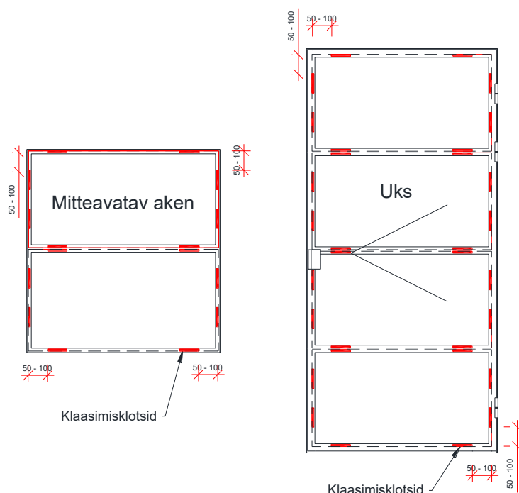
Joonis 5 Klaasimisklotside asukohad
