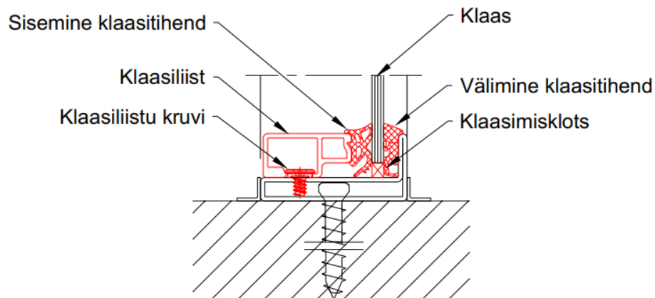
Joonis 7 Klaasi paigaldus
