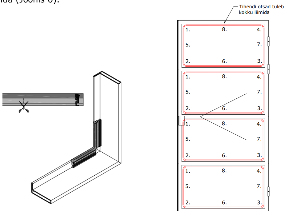
Joonis 6 Välimise klaasitihendi paigaldus
