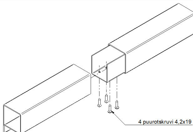
Joonis 12 Raami koostamine kasutades juhtdetaile
