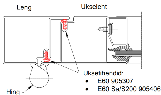
Joonis 4 Uksetihendite paigaldus
