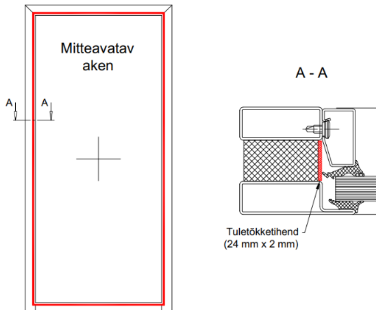
Joonis 7 24 x 2 mm tuletõkketihendi paigaldus
