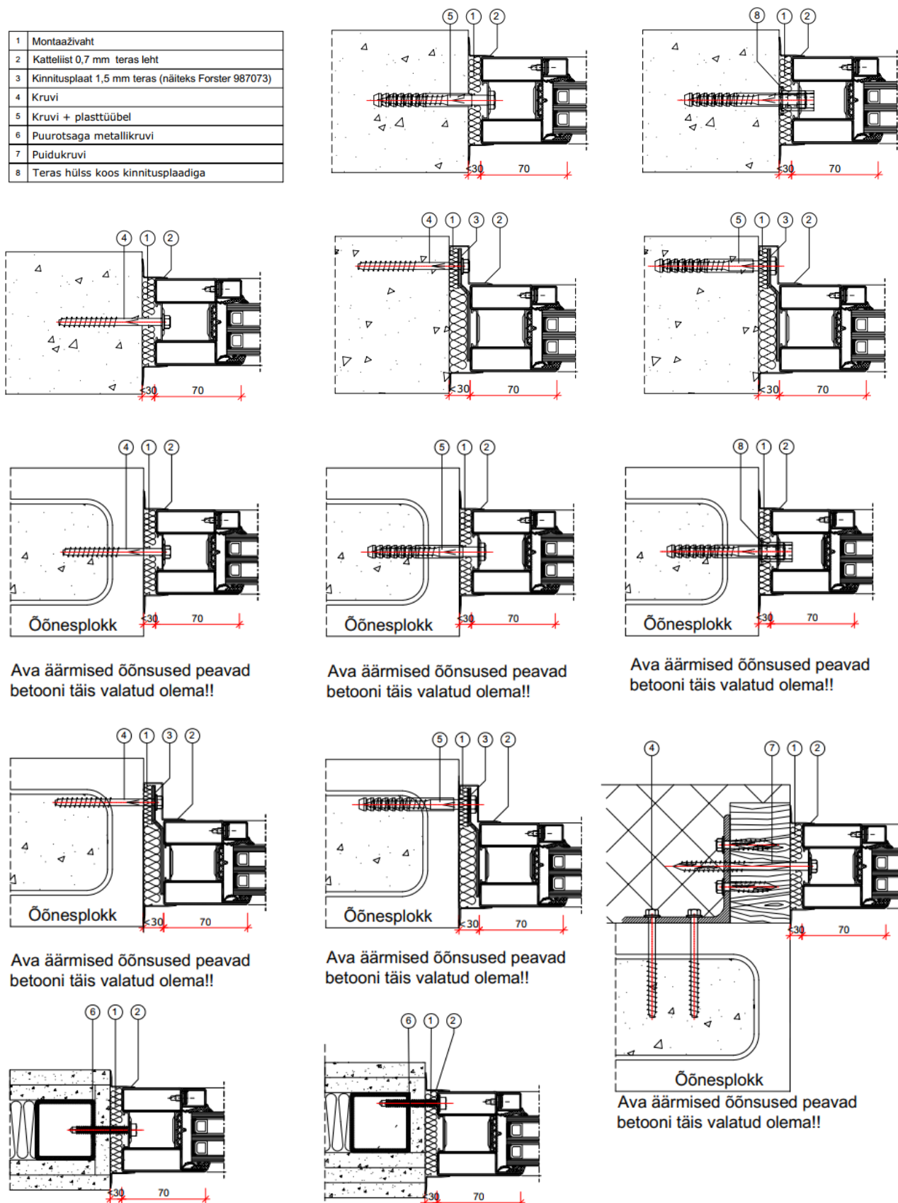
Joonis 1 Seinakinnitused vastavalt seinatüüpidele
