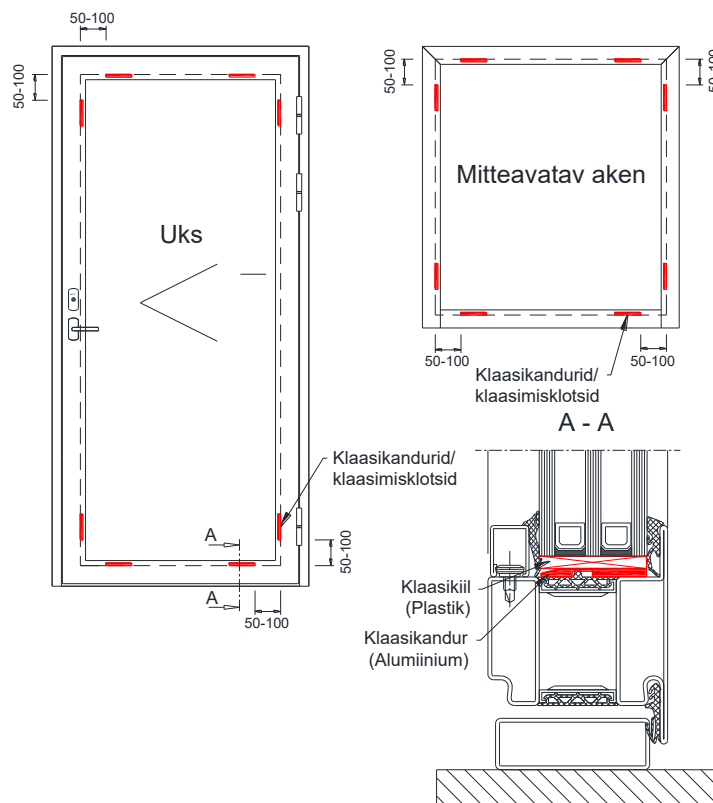
Joonis 12 Klaasimisklotside asukohad
